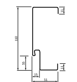
Rysunek techniczny
