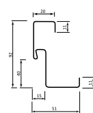
Rysunek techniczny
